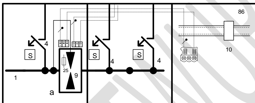
Abb. 4: Netzseitiger Anschlussraum mit Spannungsversorgung aus SPD Typ 1
